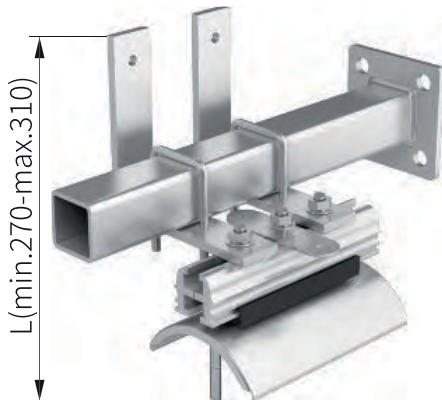
Технические характеристики тянущей тележки
